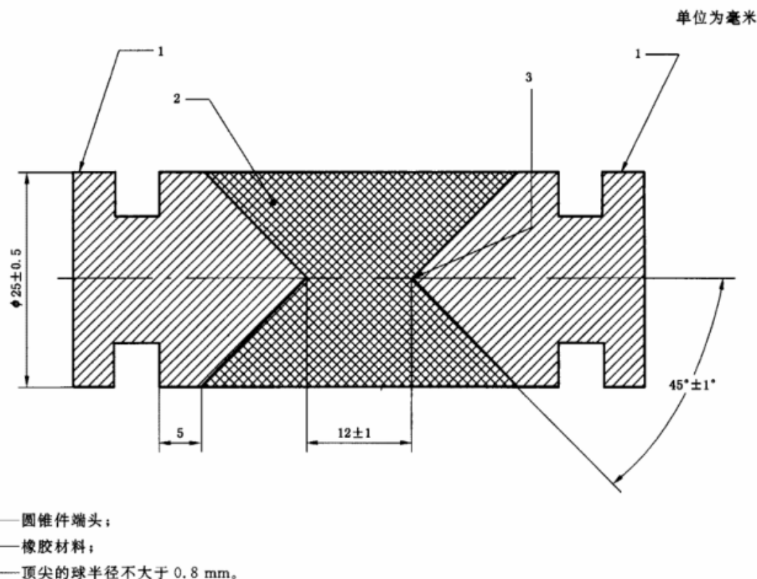
图 1 标准试样
